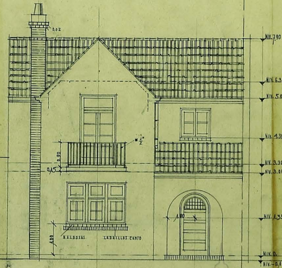
ELEVACION NORTE
