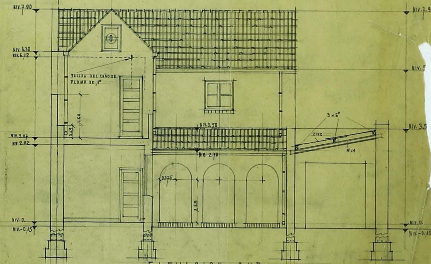
ELEVACION SUD
