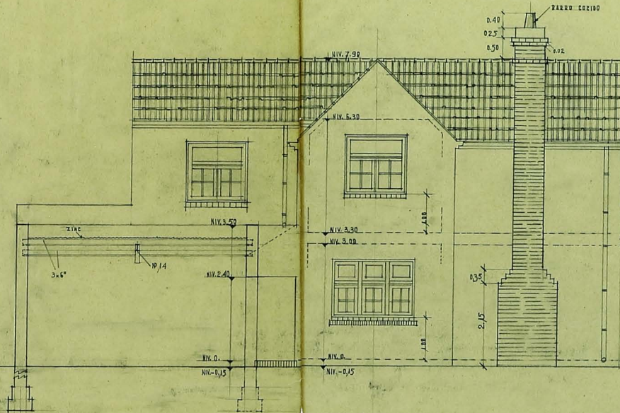
ELEVACION ESTE
