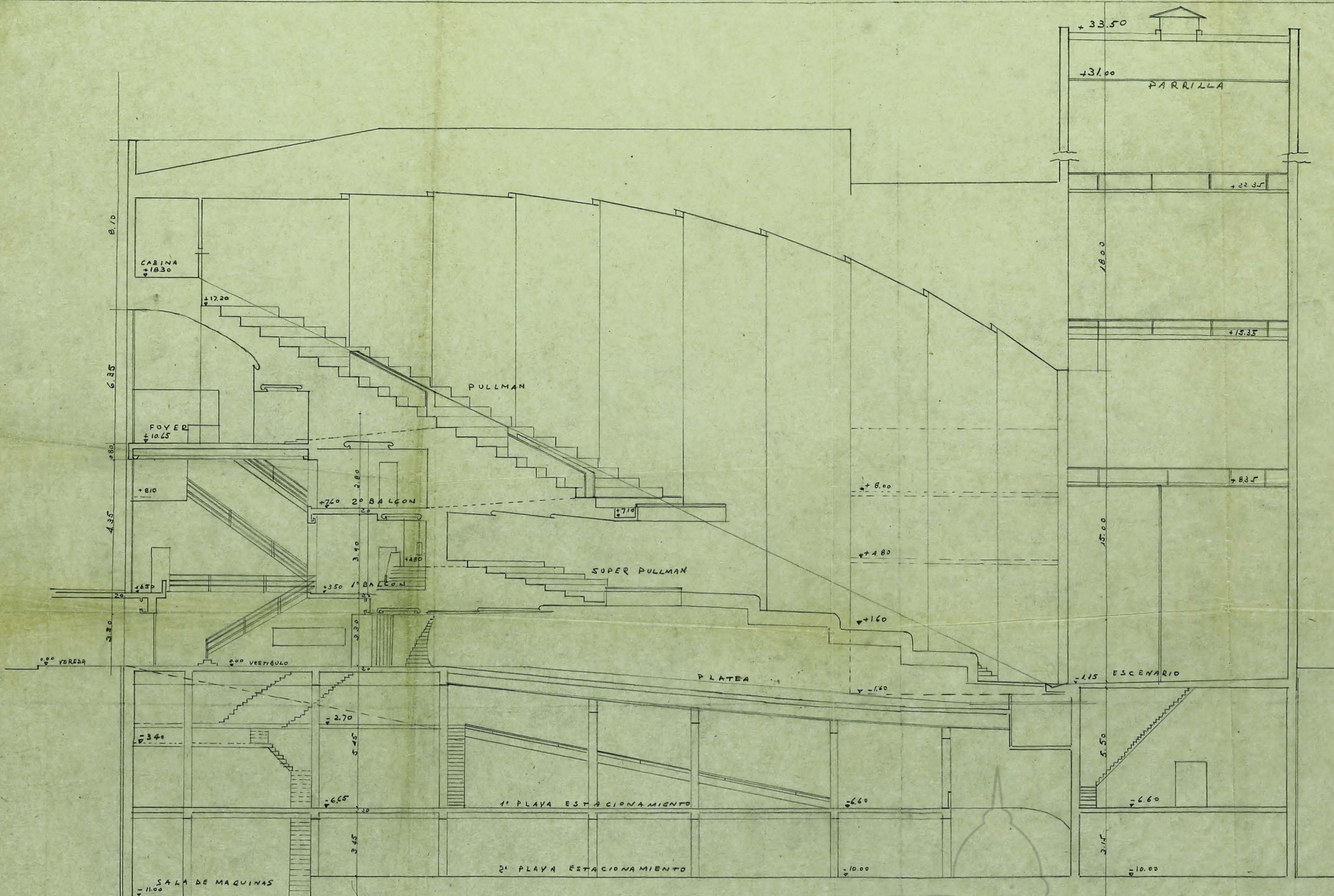
CORTE LONGITUDINAL
