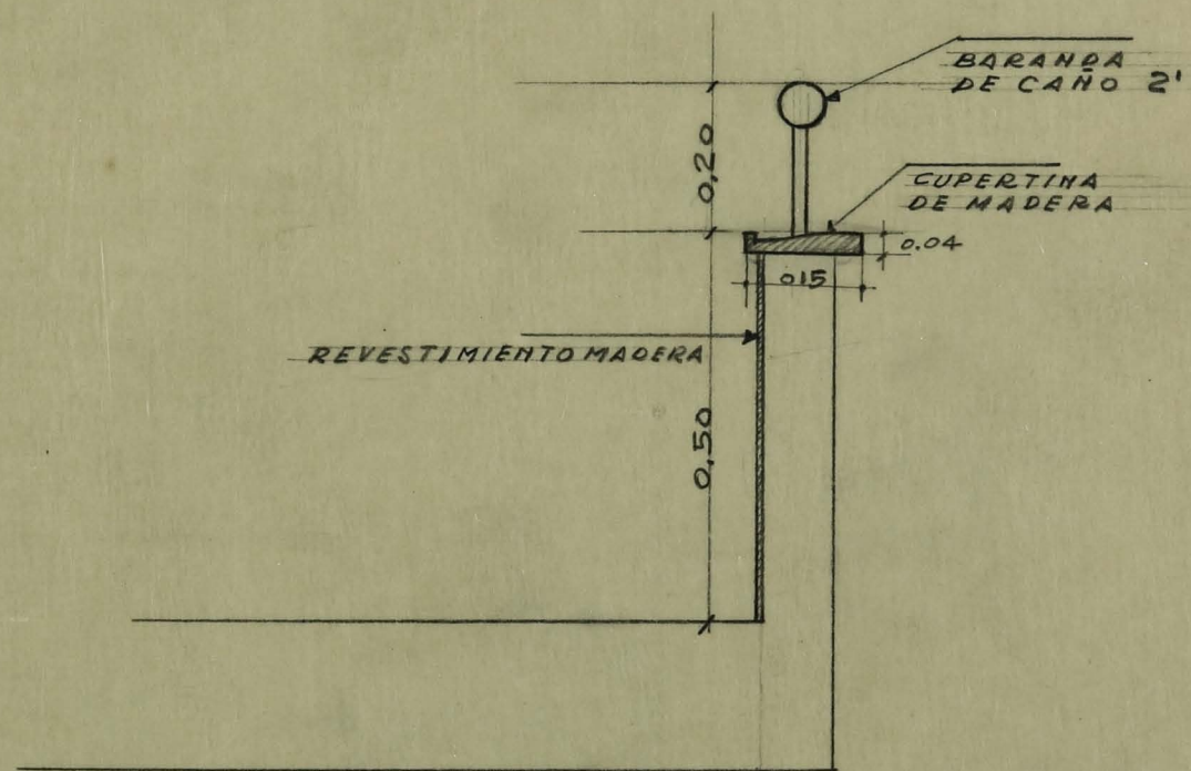
CORTE A-B.
