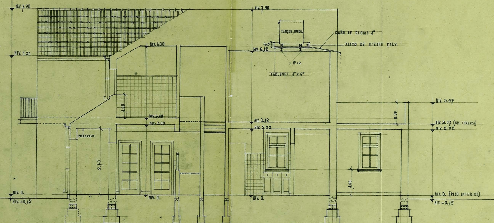
SECCION A-B
