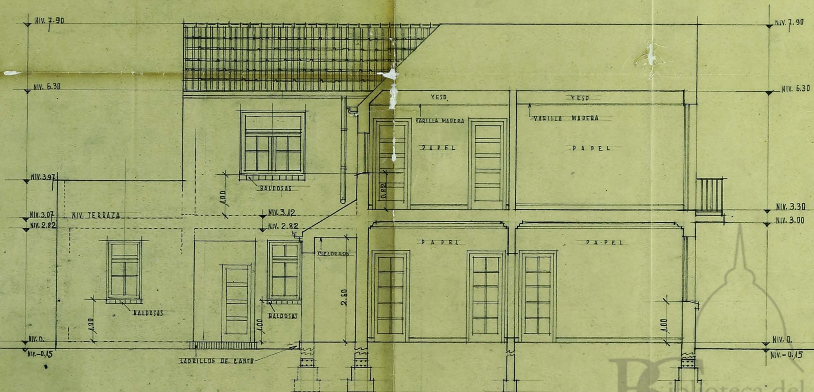
SECCION C-D
