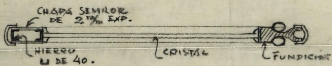
SECCION TRANSVERSAL
