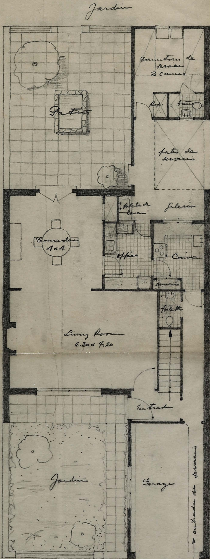
Planta baja
