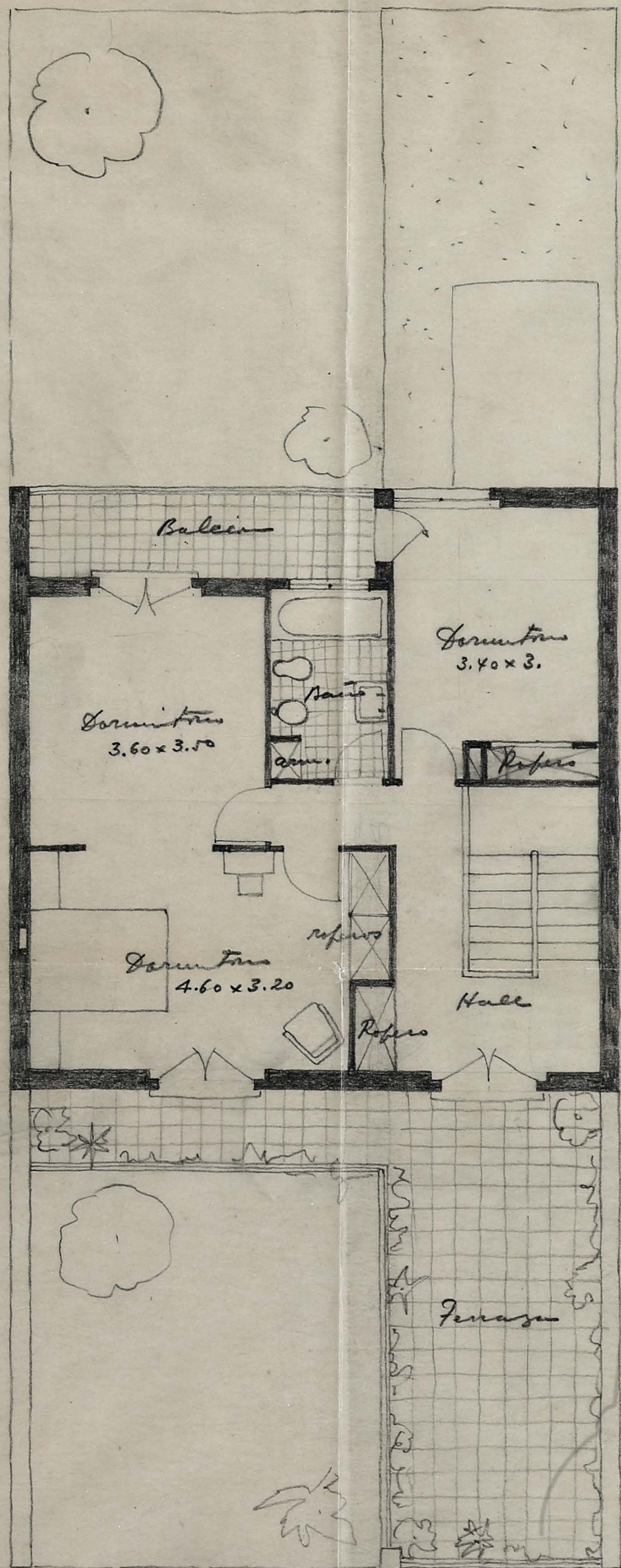
Planta alta
