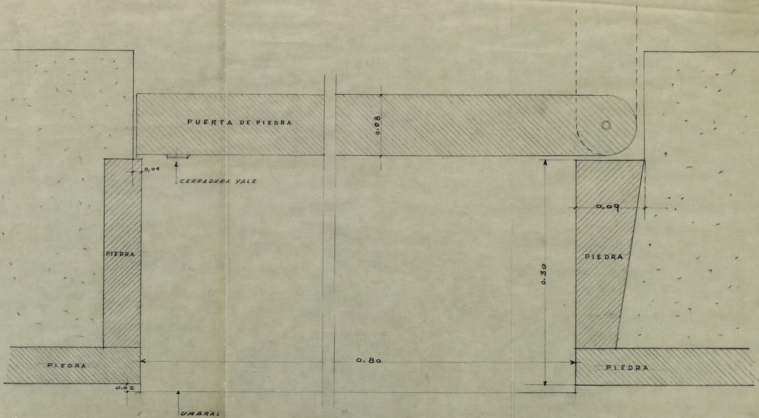
SECCION A-B
