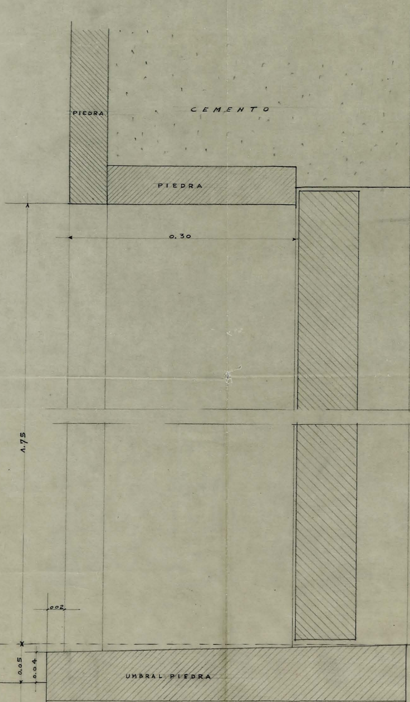
SECCION C-D
