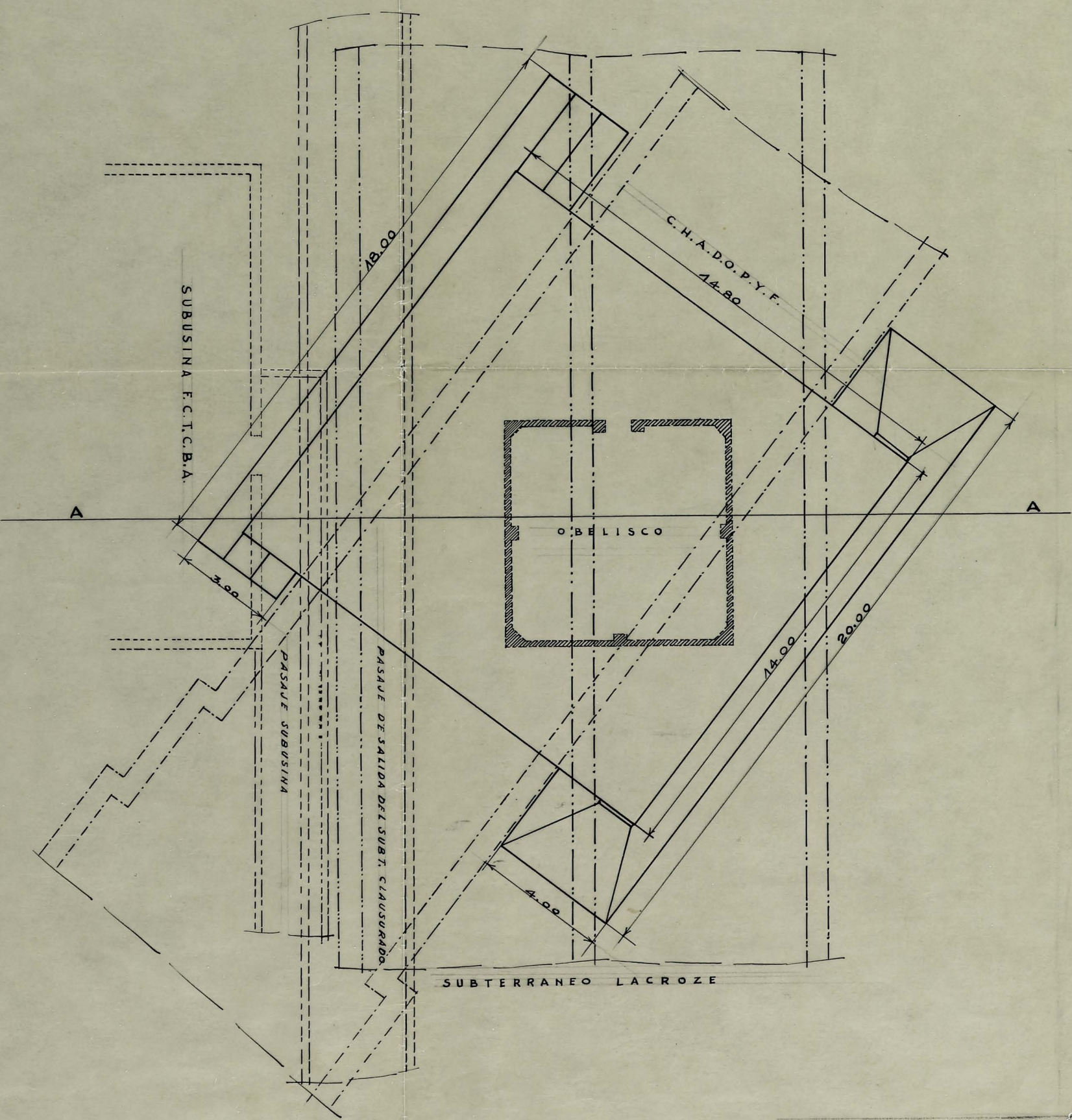
Plano definitivo de fundaciones
