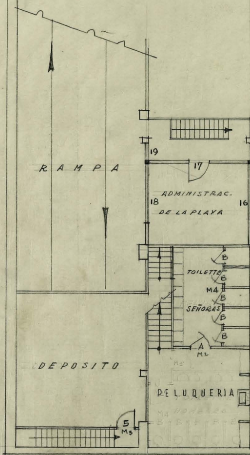
PLANTA ENTREPISO ESCALA 1:100
