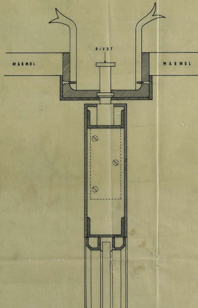
SECCION A-B
