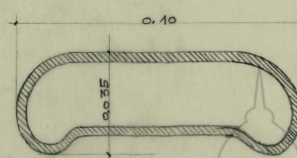
SECCION C-C TIPO GENERAL DE PASAMANOS
