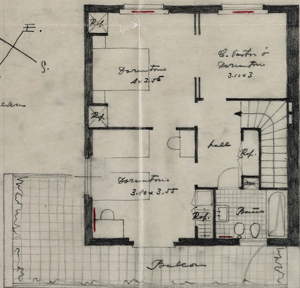
Planta Alta
