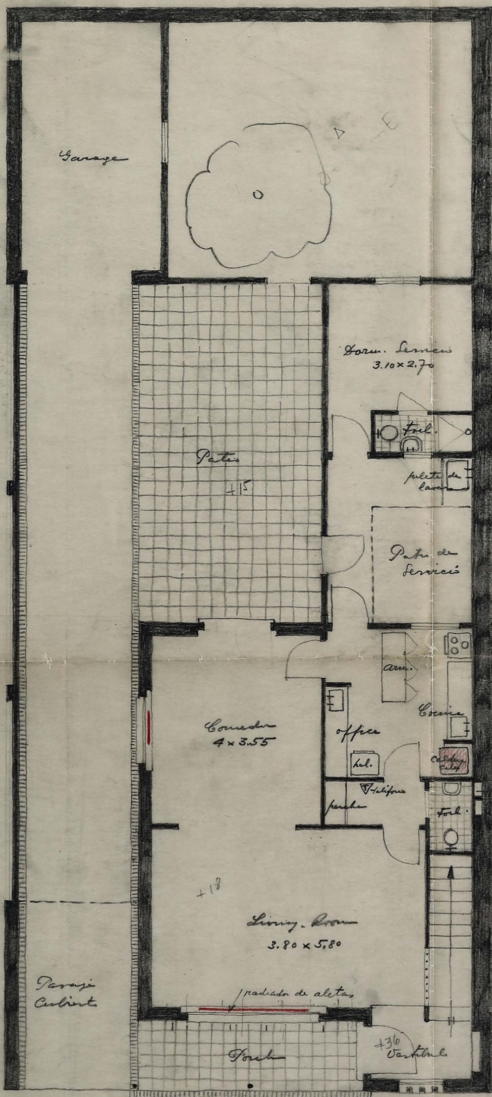
Planta Baja
